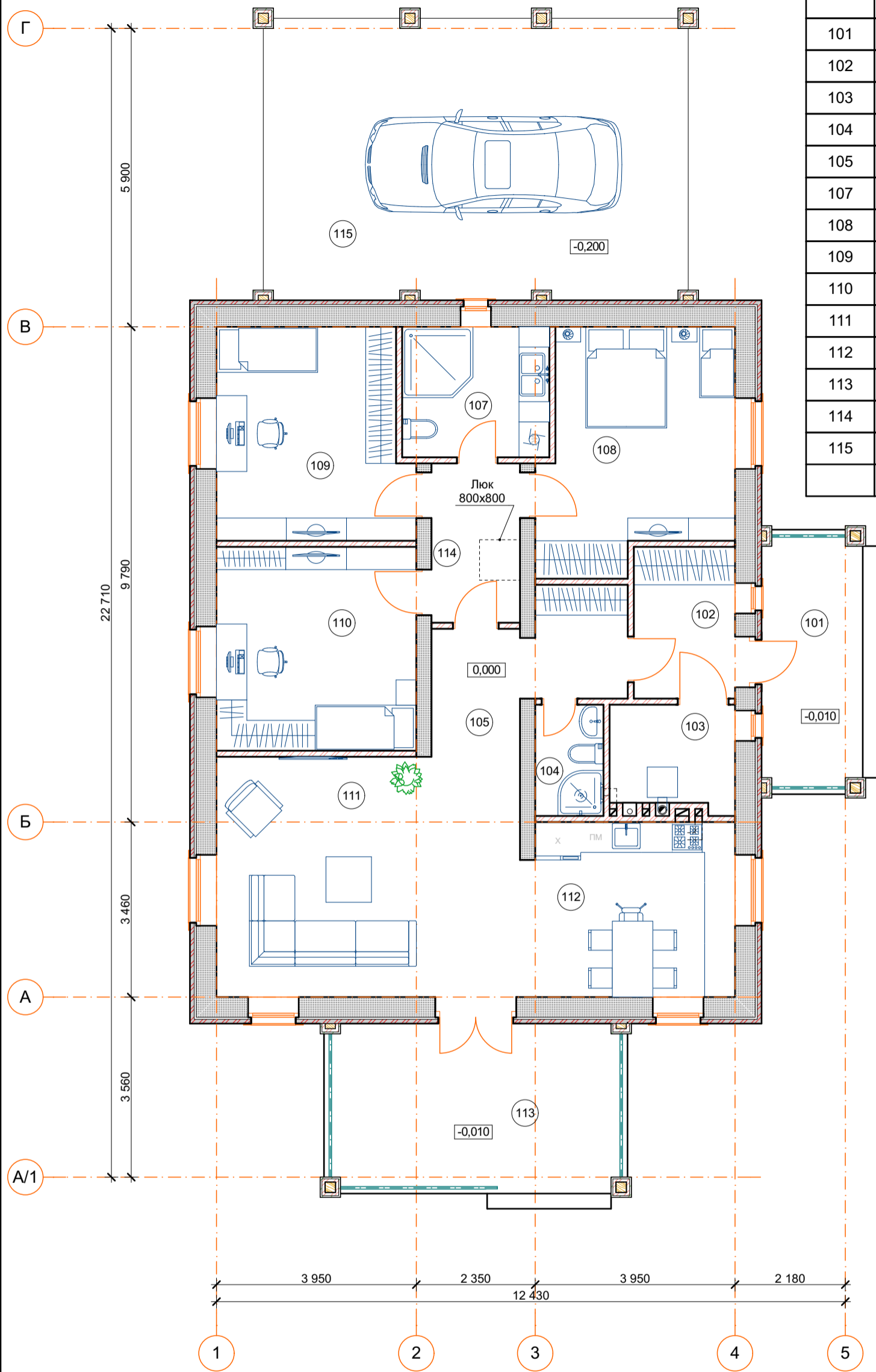
План 1-го этажа
